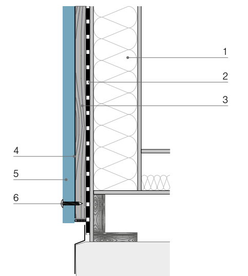
Abb. Schnitt J-J Unterer Teil der Wand
