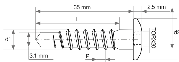
Abb. Torx-Befestigungsschraube - Aufbau und Abmessungen
