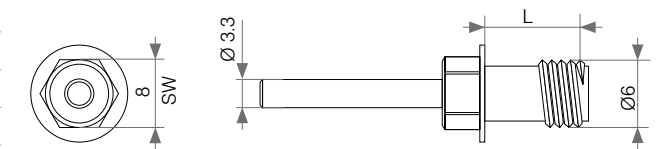
Abb. Nietschraube TU-S6,0x9 - Konstruktion und Abmessungen (mm)(mm).
