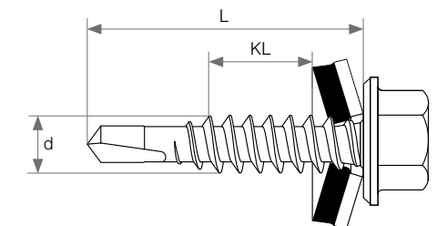
Abb. Selbstbohrender Verbinder - Aufbau
