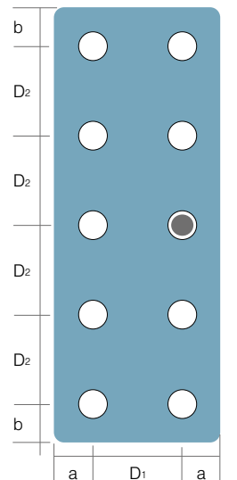
Fig. Einfeld-Befestigung
