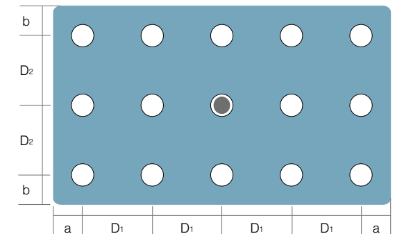
Fig. Verteilung der Verbindungen - Mehrfeld Befestigung
