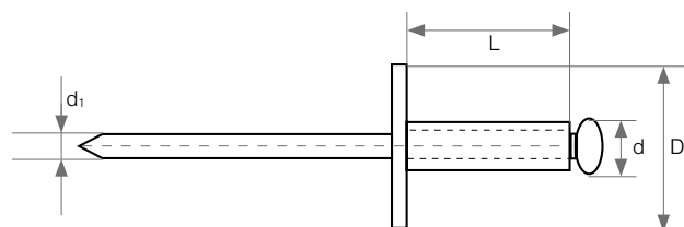
Abb. Einfacher Niet - Konstruktion und Abmessungens
