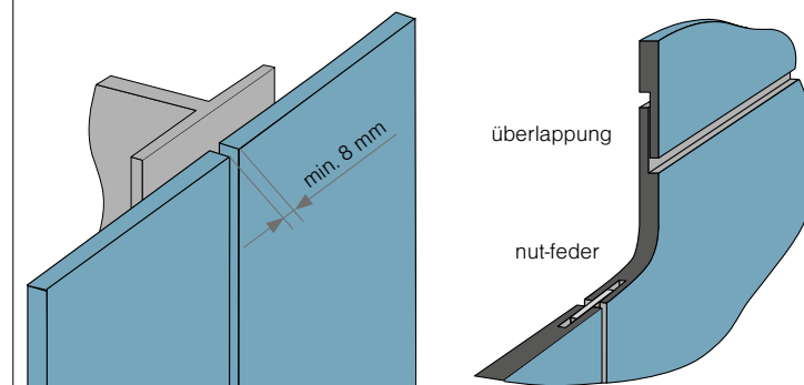
Abb. Offenes Fugensystem
