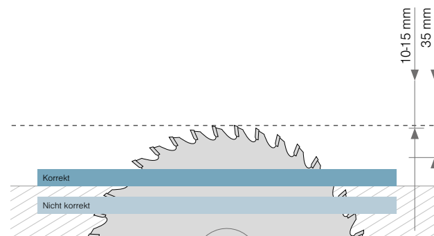
Abb. Kreissäge, positiver Eintrittswinkel des Sägeblatts, Sägegasse unter dem Werkstück
