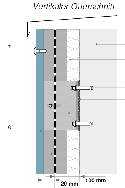
Abb. Schnitt F-F Oberer Teil der Wand mit Abschlussrahmen
