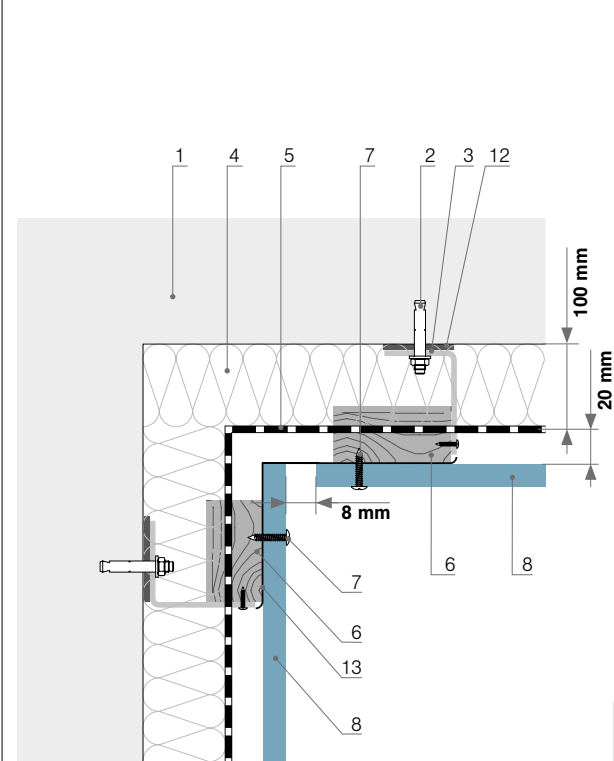
Abb. Schnitt H-H Verbindungsstück an der inneren Ecke
