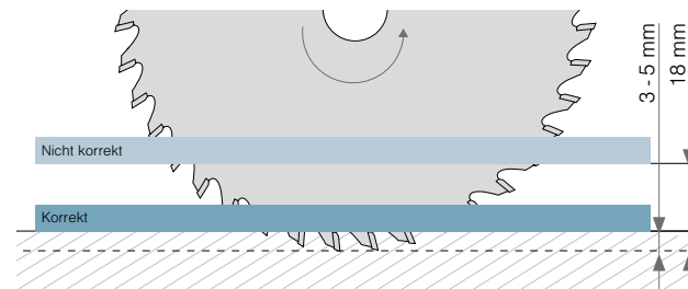
Abb. Kreissäge, negativer Eintrittswinkel des Sägeblatts, Sägegasse über dem Werkstück
