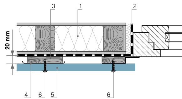
Abb. Schnitt C-C Verbindungsstück mit Fensterelementen (innen)
