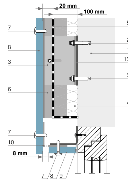
FAbb. Schnitt D-D Verbindungsstück mit Fensterelement (innen)
