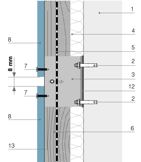
Abb. Schnitt B-B Profil-Verbindungsstück
