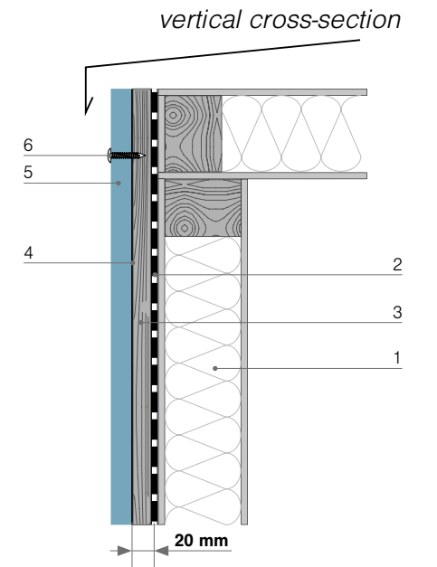
Abb. Schnitt F-F Oberer Teil der Wand mit Abschlussrahmen
